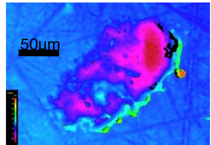
Abbildung 2 – Höhenbild der hinterlassene Spur eines Funkens
